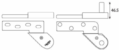
Top pivot
