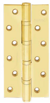
BHP 612 8"X4"X5MM 4BB 130KG/PAIR
