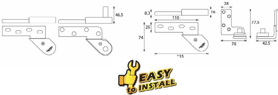
Bottom pivot
