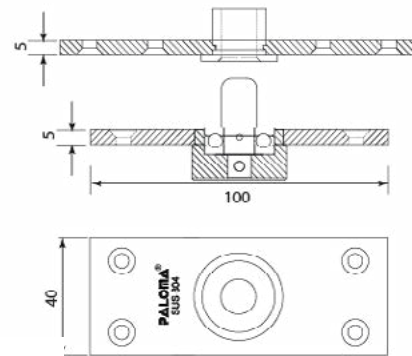
Bottom pivot
