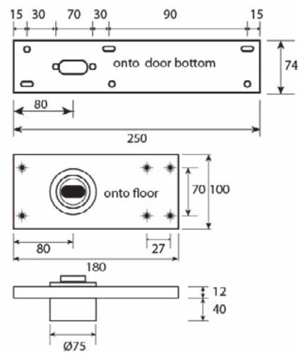
Bottom pivot
