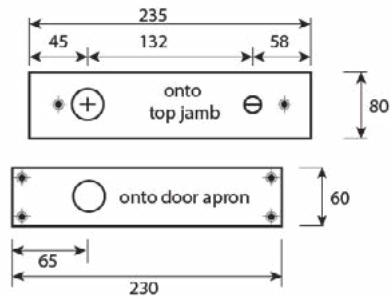
Top pivot
