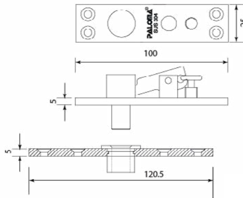
Top pivot
