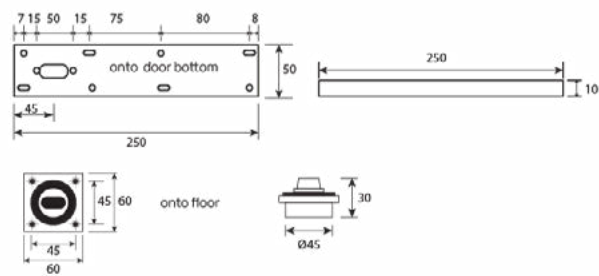
Bottom pivot
