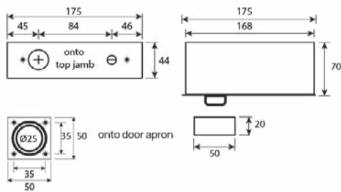
Top pivot
