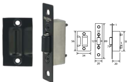
RCP 202 ROLLER CATCH PLM-500 SUS 304
