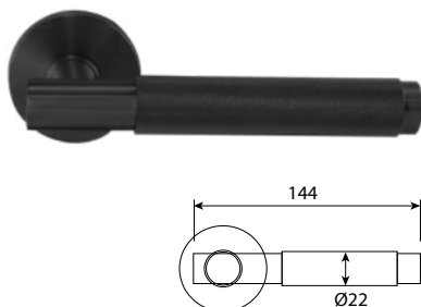
HRP 7202 HAGEN BB
