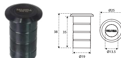
DPP 202 DUST PROOF SUS 304
