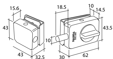
GLP 2102 G/G SS 2100
