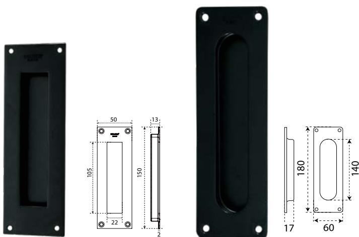
CMP 221 SQUARE 15CM
