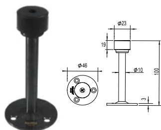
DSP 222 WALL 013 SUS 304
