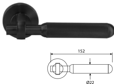
HRP 7152 SOFIA BB
