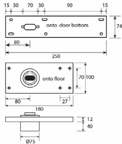
Bottom pivot
