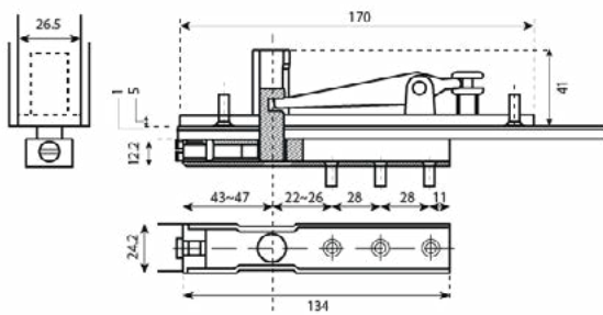
Top pivot
