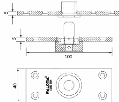
Bottom pivot
