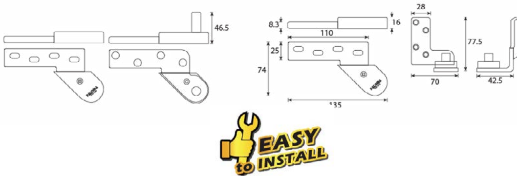
Bottom pivot
