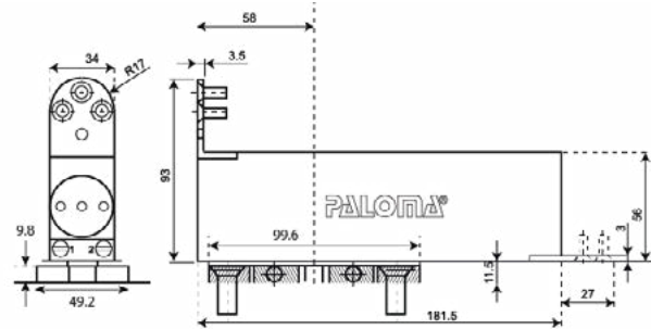
Bottom pivot
