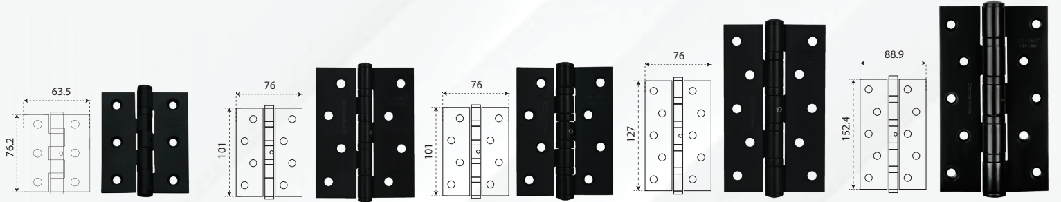
BHP 231 3"X2.5"X2MM 2BB NRP SUS 304 - MAX 40KG / PAIR
