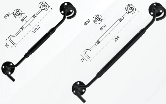
WHP 657 603-8" BL - BRASS
